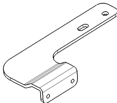
后固定支架 LH Rear fixed bracket LH 数量 QTY: 1
